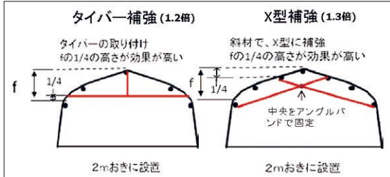
▲図1 タイバー、X型補強
